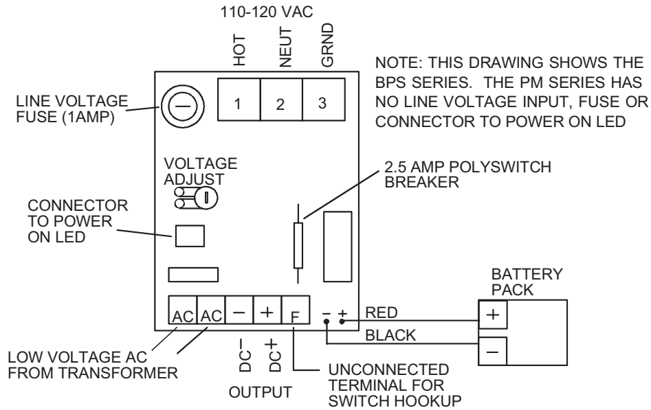
FIG. 2: WIRING
